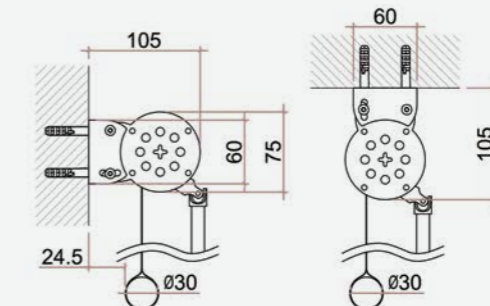
Applicazione a parete (standard)
