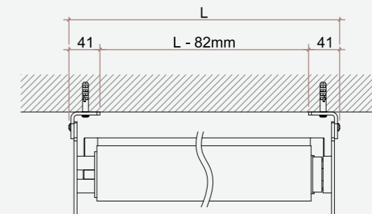
Applicazione a parete (vista dall'alto)
