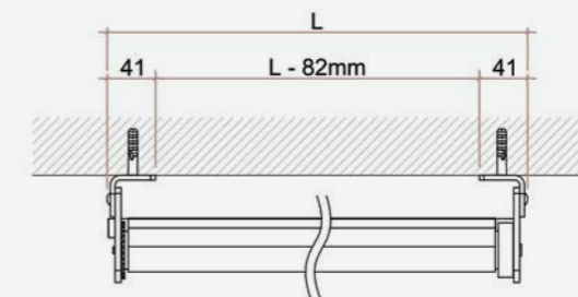
Applicazione a parete (vista dall'alto)
