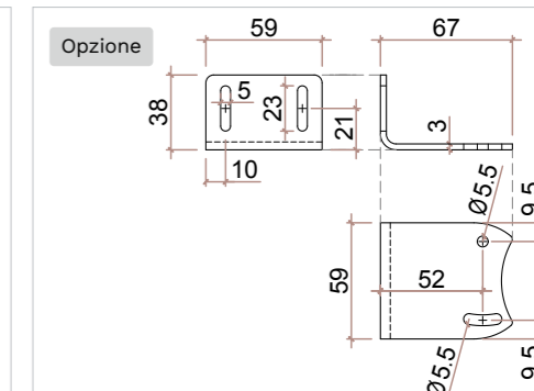
Ingombro staffa lunga
