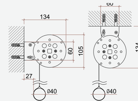
Applicazione a parete (standard)
