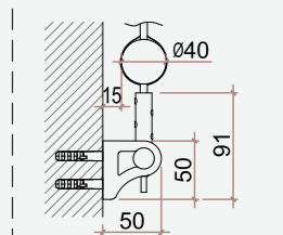
Staffa corta (opzione)
