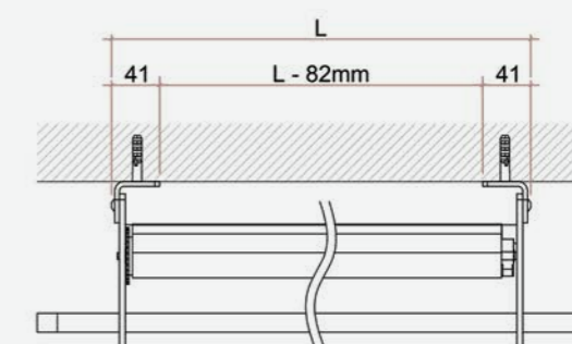
Applicazione a parete (vista dall'alto)
