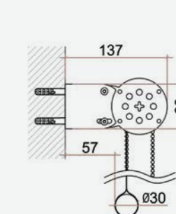
Staffa lunga per testata (opzione)
