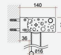
Applicazione a parete (standard)
