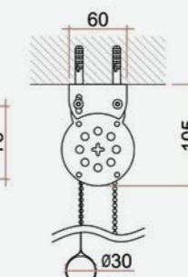
Applicazione a soffitto (opzione)
