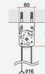
Applicazione a soffitto (opzione)
