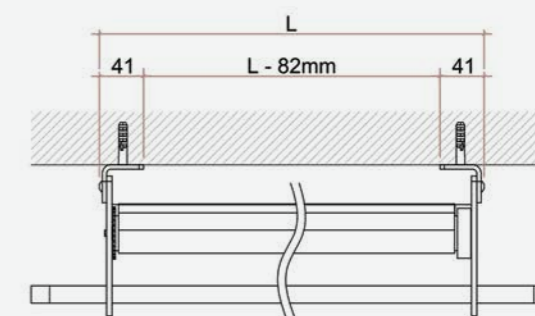
Applicazione a parete (vista dall'alto)
