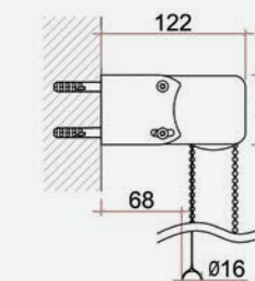
Staffa lunga per testata (opzione)
