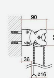
Applicazione a parete (standard)
