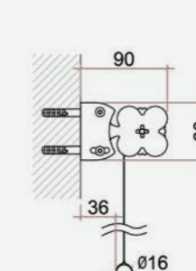
Applicazione a parete (standard)
