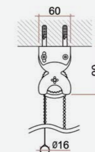
Applicazione a soffitto (opzione)
