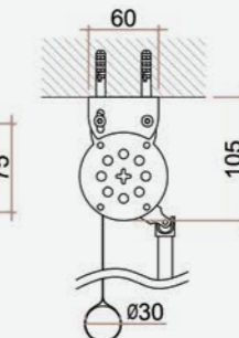
Applicazione a soffitto (opzione)
