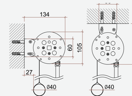
Applicazione a parete (vista dall'alto)
