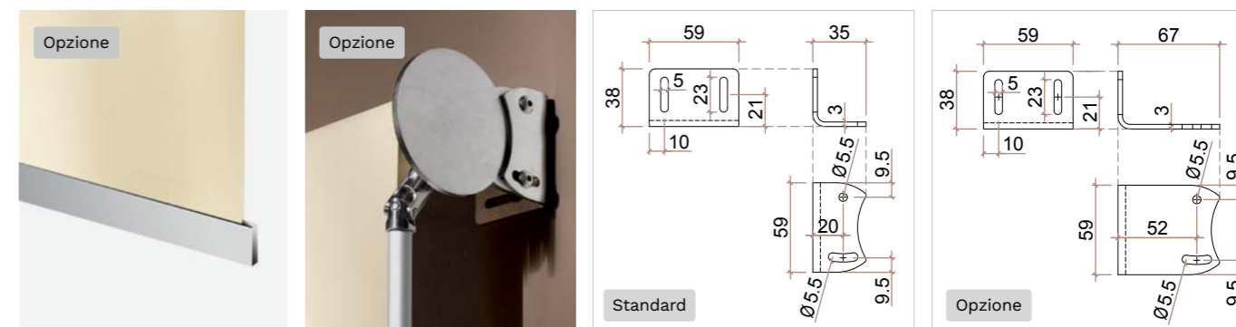
Fondale a vista
