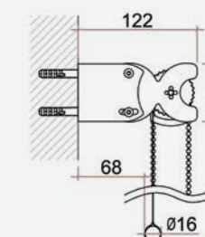
Staffa lunga per testata (opzione)
