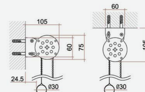
Applicazione a parete (standard)
