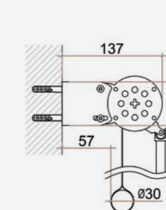
Staffa lunga per testata (opzione)
