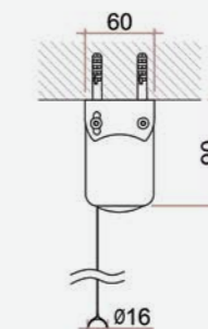
Applicazione a soffitto (opzione)
