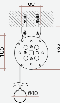
Applicazione a soffitto (opzione)
