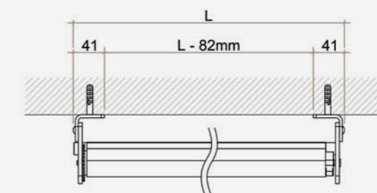
Applicazione a parete (vista dall'alto)
