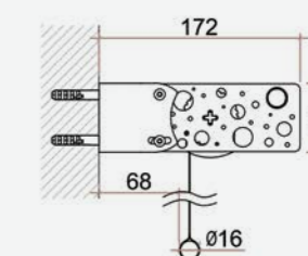
Staffa lunga per testata (opzione)
